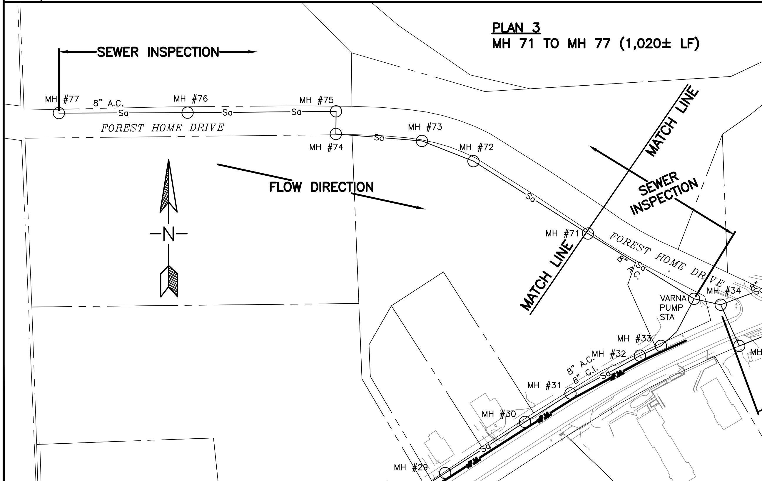
3 PLAN 3 SCALE: 1"=100'
