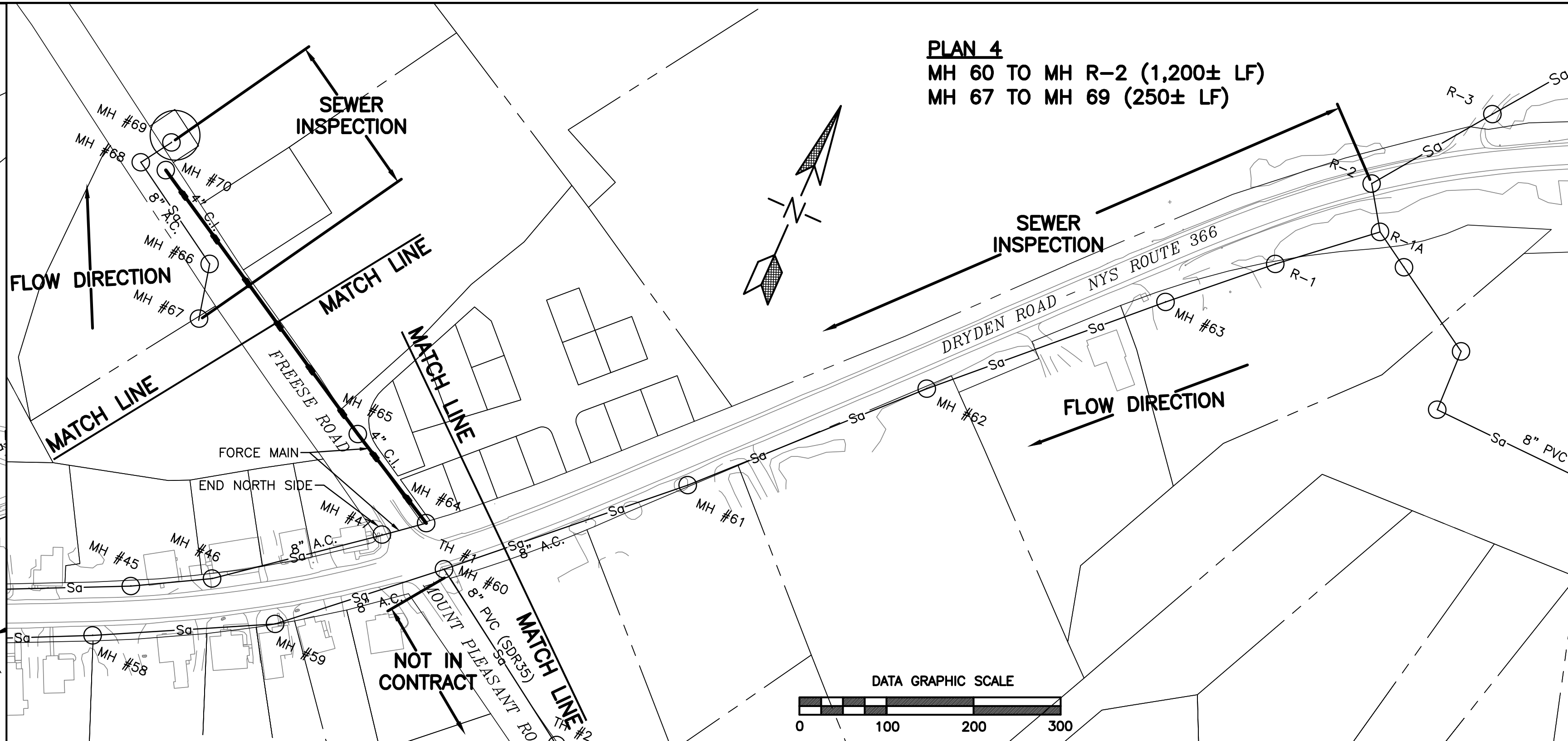
4 PLAN 4 SCALE: 1"=100'
