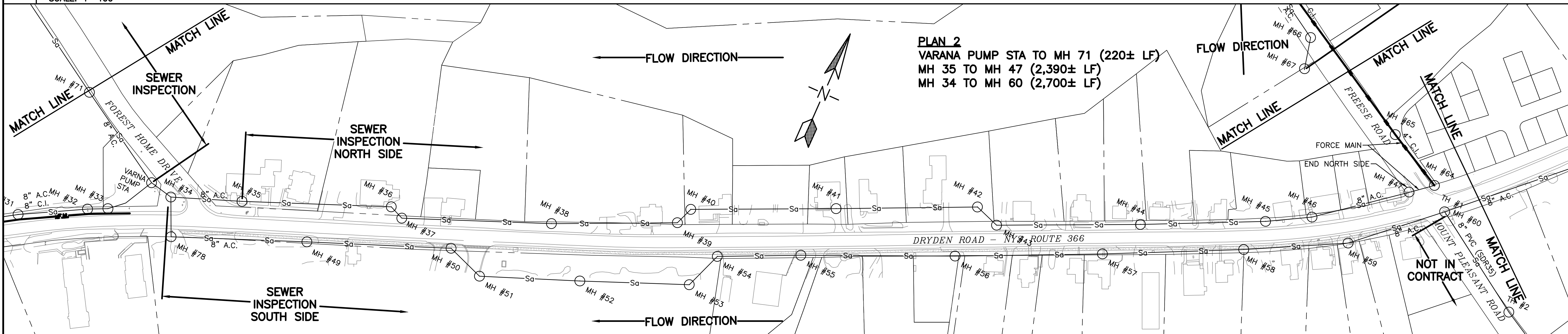
2 PLAN 2 SCALE: 1"=100'
