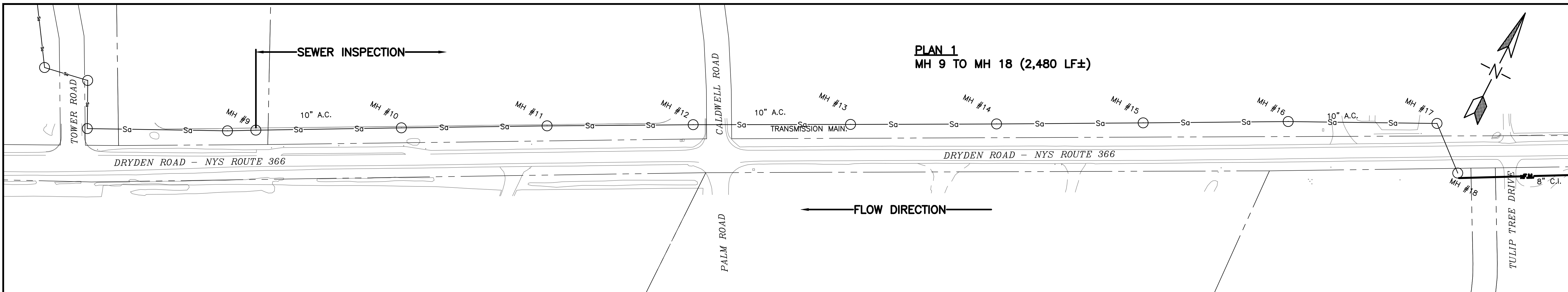
1 PLAN 1 SCALE: 1"=100'
